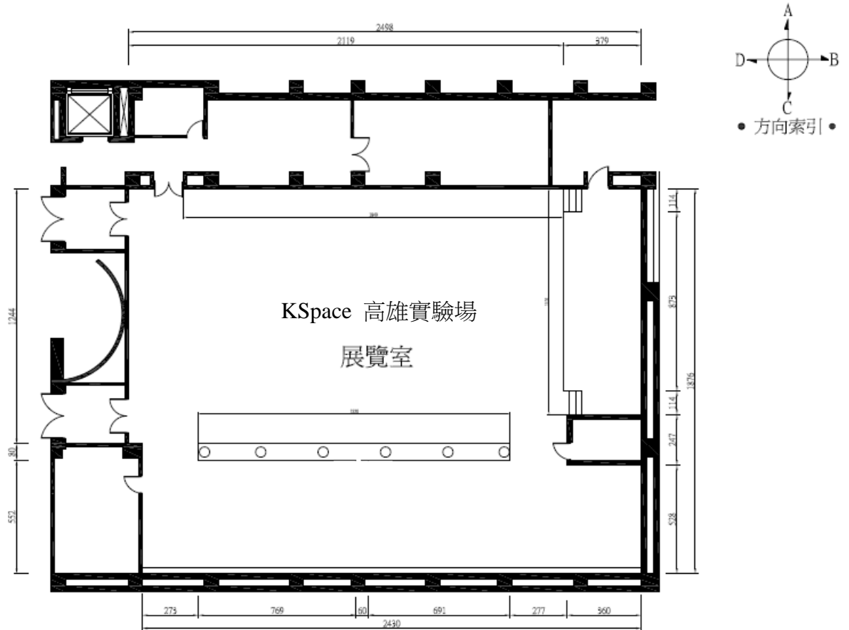
B01展覽室-平面圖 (CH:278cm) S : 1 : 150 單位：公分
