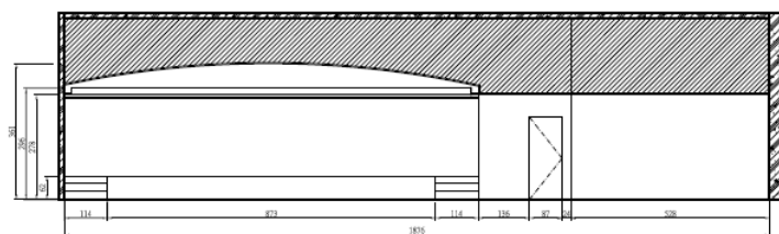
B01展覽室-B向立面圖
