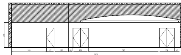
B01展覽室-D向立面圖
